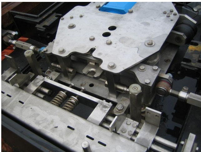
Schakel- en tongmeldmechanisme.
